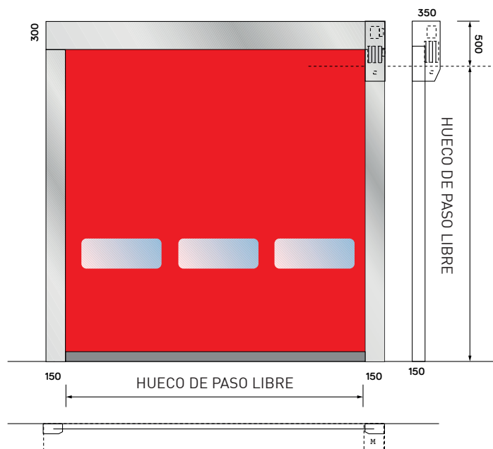
NF / AUTO ROLL MOTOR FRONTAL
