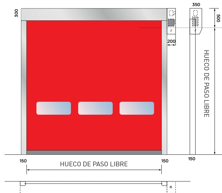
NF / AUTO ROLL MOTOR LATERAL
